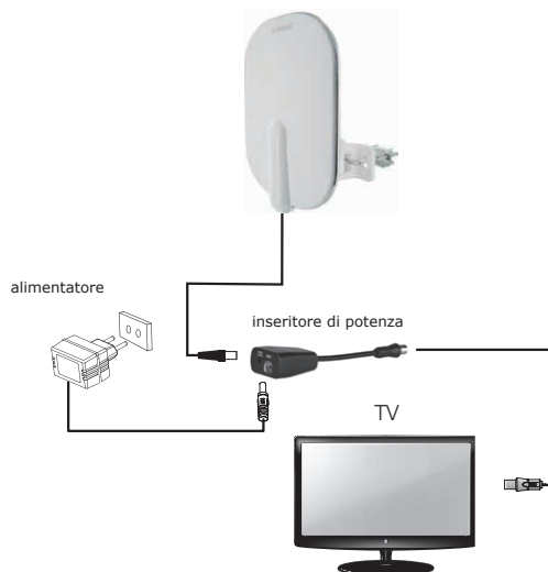
Esempio di collegamento (DESTRA)
