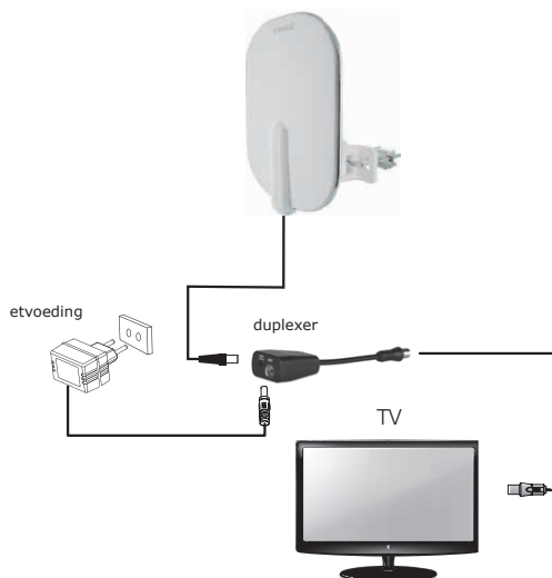
Aansluitvoorbeeld (RECHTS)
