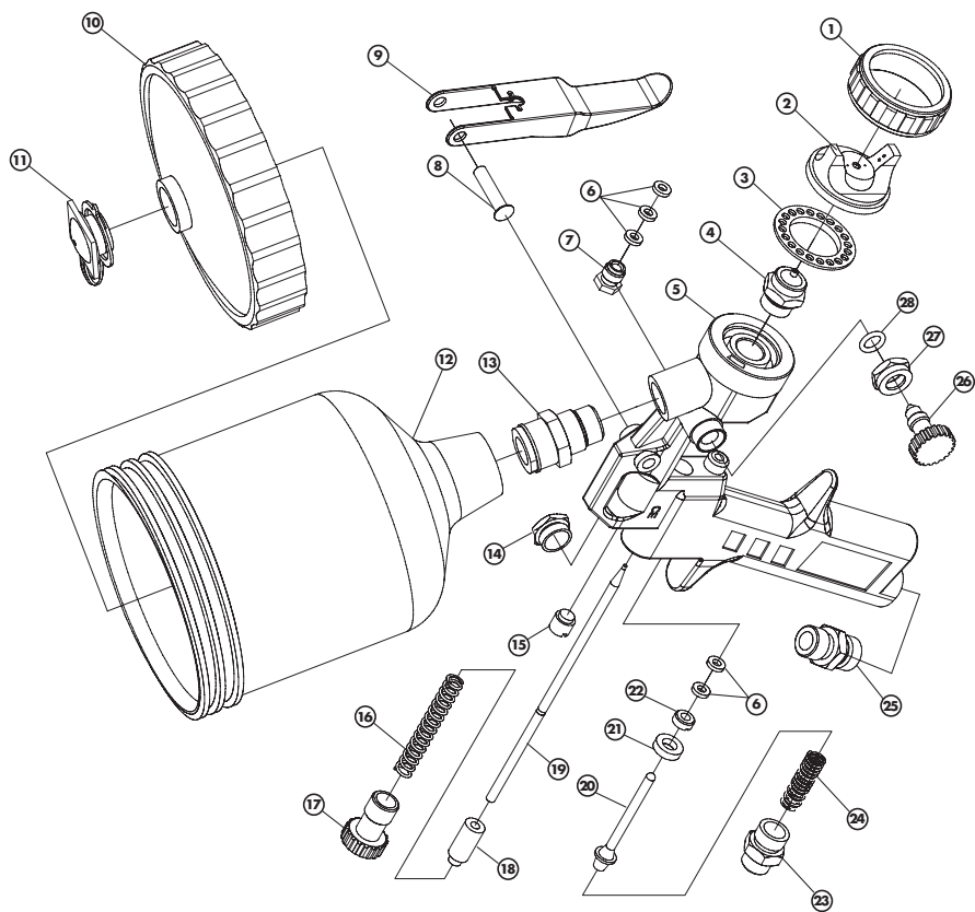
Abb. 3: Explosionszeichnung
